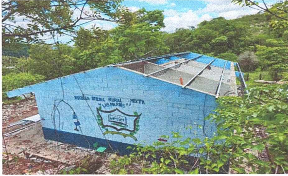
Foto1: SUSTITUCIÓN TECHO CON DURALITA Y ESTRUCTURA DE METAL POR LÁMINA TROQUELADA EN MODULO DE AULAS
