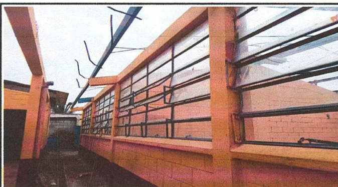
Foto 4: Arreglo de techo de corredor interno
