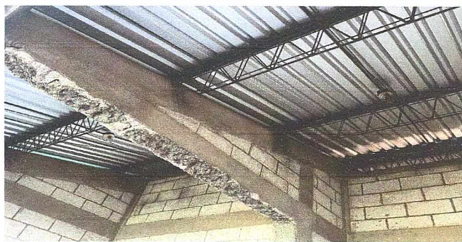
FOTO 2: Vista de techo de modulo 5 terminado.
