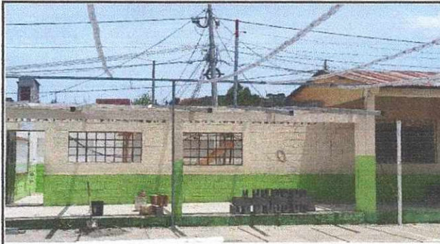
Foto 2: INSTALACIÓN DE TECHO CON ESTRUCTURA METALICA Y LAMINA TROQUELADA EN MODULO DE AULAS
