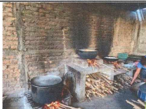
Foto 4: MANTENIMIENTO DE ESTUFA RURAL, INSTALACION DE AZULEJO, SISTEMA DE EXTRACCIÓN DE HUMO, MEJORAMIENTO DE MUEBLE DE COCINA Y PAREDES EXISTENTES EN COCINA
