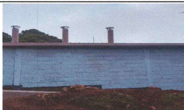
Foto 4: Sustitución de canales completo
