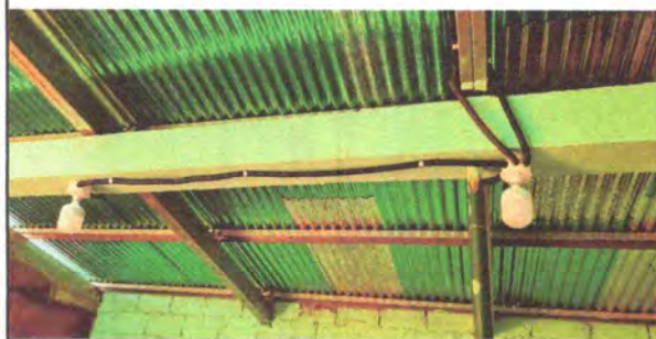
Foto 9: Sustrucción de cableado y bombillas led con interruptor
