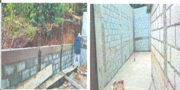
Foto 5: SUSTITUCION DE MURO DE CONTENCIÓN
