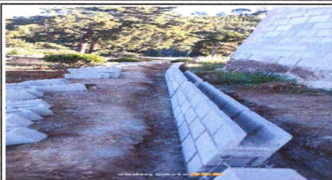
Foto 1: Reparación y mantenimiento durante el proceso de cerco perimetral con malla 200mts2
