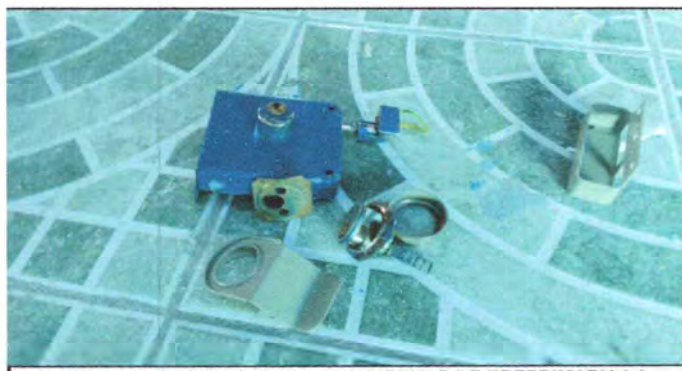
Foto 6: SE SUSTITUYE LA CHAPA DEL MODULO DE PREPRIMARIA LA CUAL TENÍA PROBLEMAS AL ABRIR.
