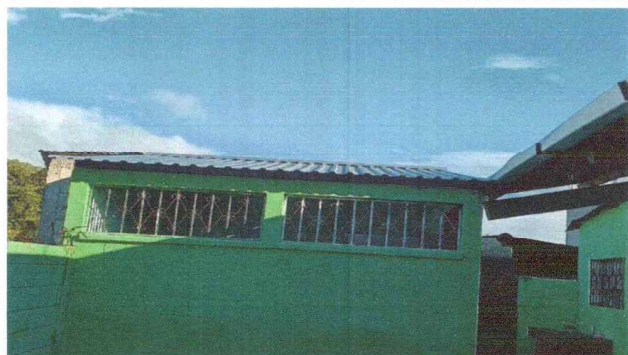
Foto 1: Cambio de costanera y lamina acanalada.
