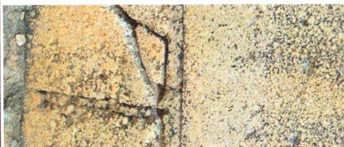
Foto4: Reparación de muro perimetral
