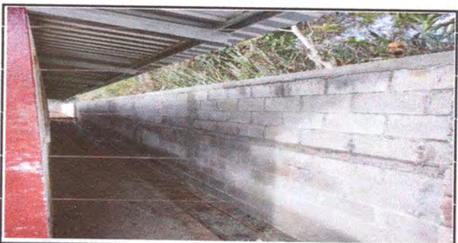
Foto: 5: suministro y reparación de muro perimetral al lado Poniente.
