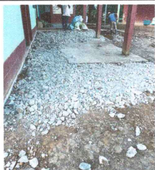
Foto 5: PREPARANDO EL TERRENO PARA LA INSTALACION DE LOSA DE CONCRETO
