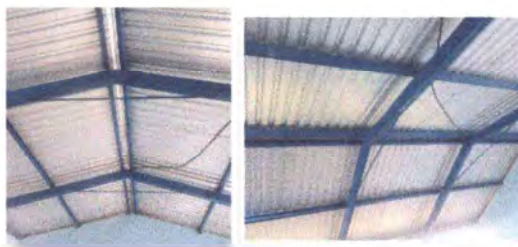
Foto 2: MANTENIMIENTO DE ESTRUCTURA METÁLICA FINALIZADO
