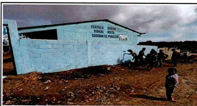
Foto 5: Se observa la finalización del muro perimetral que fue reconstruido en la Escuela por el Programa mantenimiento de Edificios Escolares Públicos.
