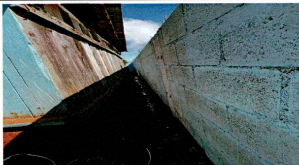
Foto 3: Se observa la reconstrucción de muro perimetral en proceso o termino medio que se realiza en la Escuela.
