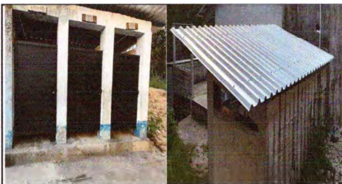
Foto 6: REPARACION DE PUERTAS DE METAL E INSTALACION DE LAMINA Y ESTRUCTURA EN SERVICIOS SANITARIOS
