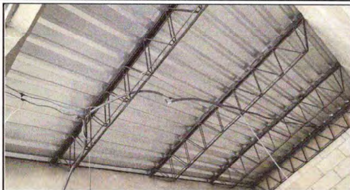
Foto1: INSTALACION DE REFUERZO DE ESTRUCTURA EN PROCESO
