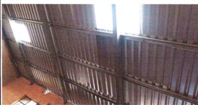
Foto: 13 Sustitución de lamina troquelada y estructura de madera por estructura de costaneras realizada en aula
