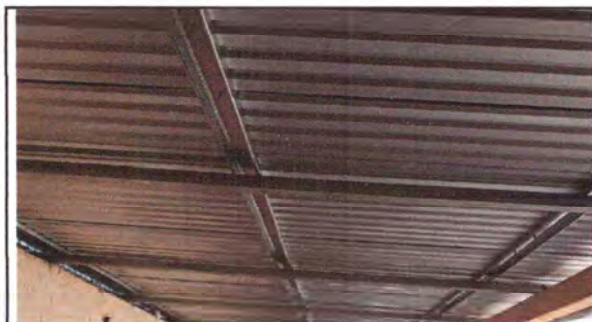
Foto: 9 Sustrucción de lamina troquelada y estructura de madera por estructura de costaneras realizada en cocina
