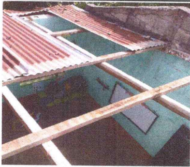
Foto 1: SUSTITUCIÓN DE LÁMINA TROQUELADA CALIBRE 26
