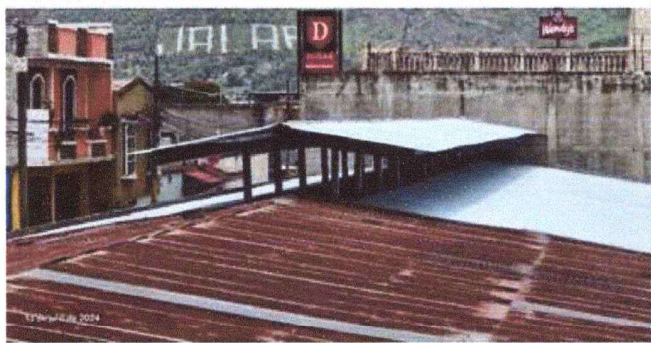
Foto1: SUSTITUCION DE LAMINA EXISTENTE POR LAMINA ACANALA CALIBRE No. 26
