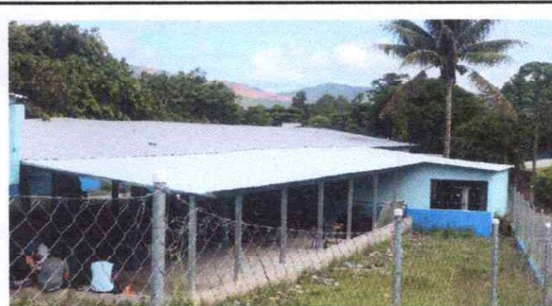
Foto 4: sustitucion de estructura de soporte de madera por metal
