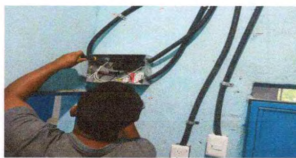
Foto 10. Sustitucion de flipones
