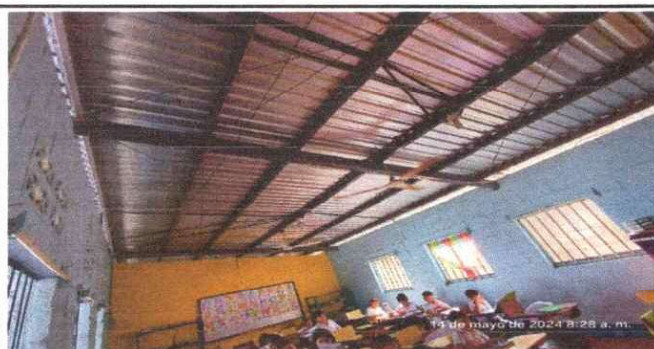
Foto 5: Sustitución de cableado eléctrico.
