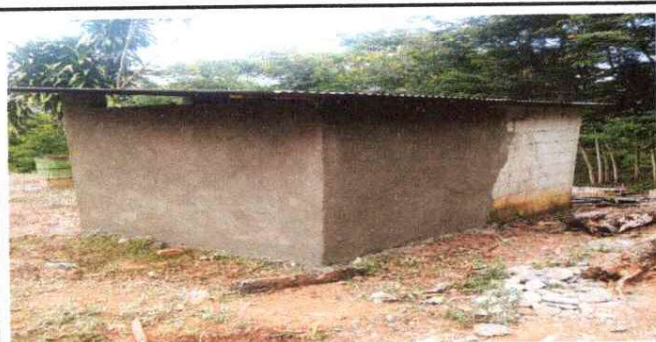
FOTO 5: PROCESO DE REPELLO EN MURO
