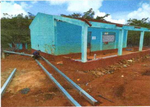
Foto 1: Sustrucion de estructura de madera por estructura metalica
