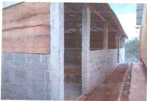
FOTO 1: Se observa la construcción de dos aulas nuevas con el revoque
