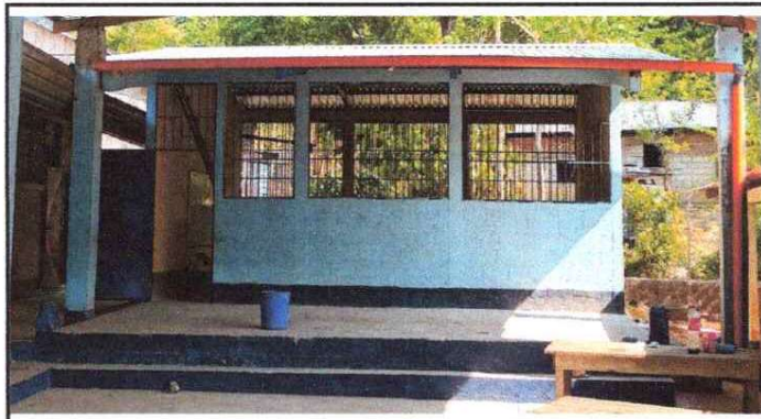
FOTO 2: FABRICACIÓN E INSTALACIÓN DE ESTRUCTURAS METALICAS, INSTALACIÓN DE LAMINAS TROQUELADAS.
