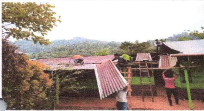
FOTO 1: Desmontaje de laminas acanaladas.
