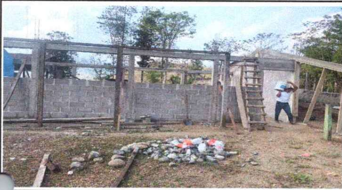
FOTO 1: REMODELACIÓN Y LEVANTAMIENTO DE MURO DE AULA.
