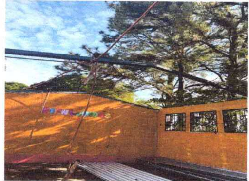
Foto 2. Sustitución de lámina, por lamina troquelada aluzinc calibre 26
