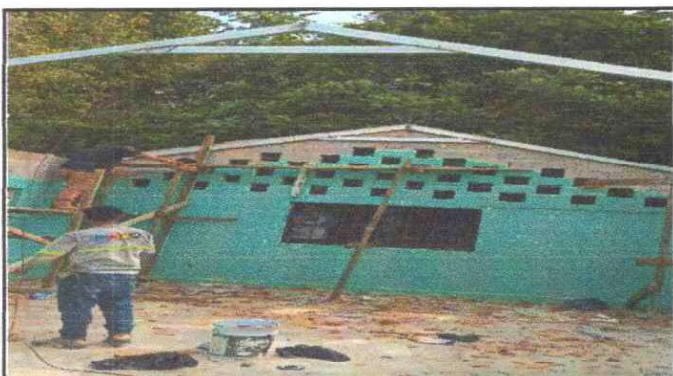
instalando la estructura metalica en los salones de cuarto y sexto primaria.
