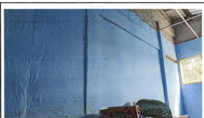
Foto 9: AMPLIACION MURO EN AULA CON REFUERZO ESTRUCTURAL PAREDES CON TABLAYESO SOBREPUESTO
