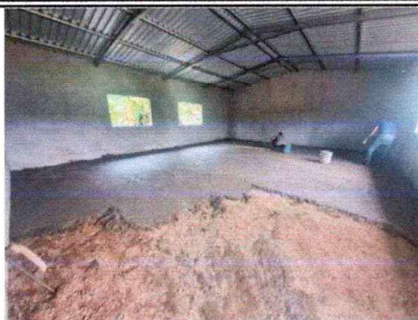
Foto 7: Suministro e instalación de piso plancha de concreto
