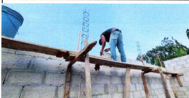
Foto 3: Suministro y levantado de block, Soleras y columnas.
