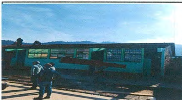
Foto1: Quitando la lámina en mal estado y dejando todo preparado para la colocación de la lámina nueva.
