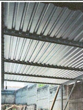
Foto 1: Cubierta de lámina: sustitución de lámina troquelada aluzinc calibre 26 y estructura de techo
