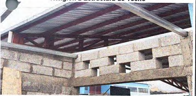
Foto 5: Se inicia el trabajo con el cambio de la estructura del techo
