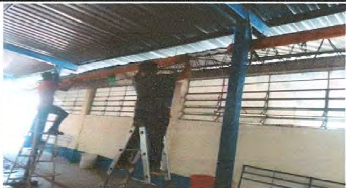
Foto1: Cambiando bajada de agua
