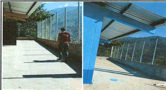
Foto 13: Sustitución de muro perimetral de block con tubo hg y malla galvanizada, soleras intermedias y columnas.
