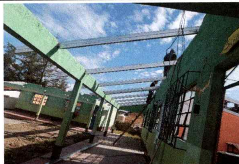
Foto 2: Sustitución de costanera de madera por tubos de metal
