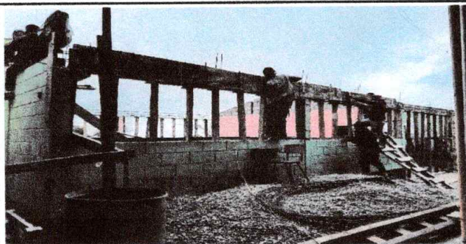
Foto 3: REPRCIÓN DE VIGA CORONA
