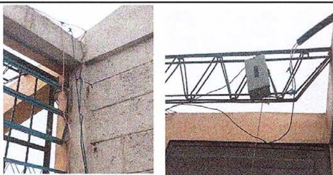
Foto 11: Sustitución de cable THH 100 AWG
