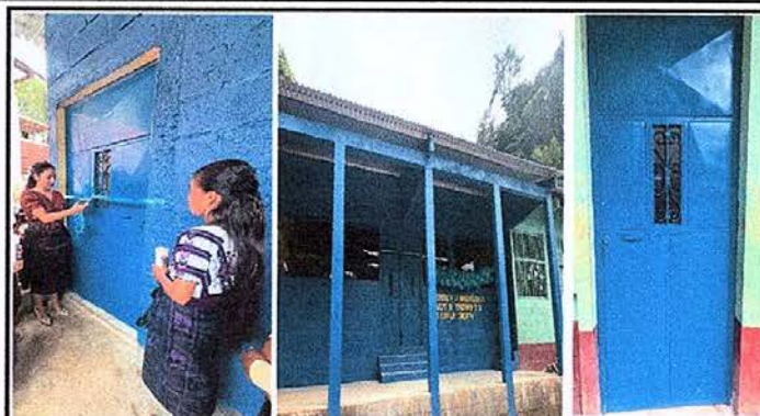
Foto 2: Sustitución de 4 puertas metálicas de ancho 1.00 mts por 2.10 mts en cocina y aulas.
