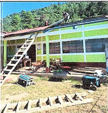
Foto 1: Sustitución de cubierta de lámina.
