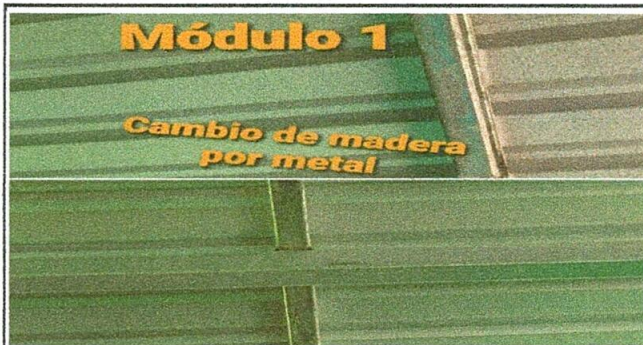
FOTO 4 SUSTITUCIÓN SOPORTE ESTRUCTURA MADERA POR METAL
