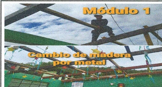
FOTO 4 SUSTITUCIÓN SOPORTE ESTRUCTURA MADERA POR METAL
