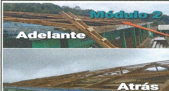
FOTO 2 SUSTITUCIÓN DE LÁMINA MÓDULO 2
