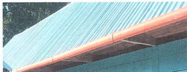
Foto 6: Sustitución de canales de agua pluvial de PVC
