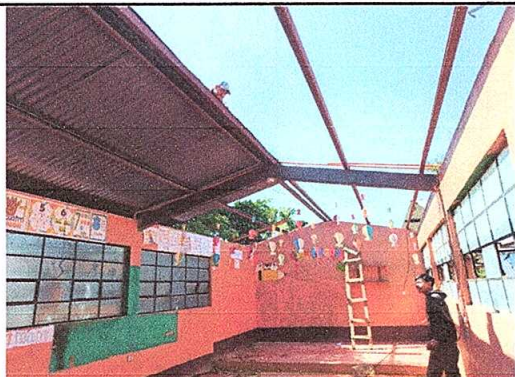
Foto 1: Sustitución de cubierta de lámina.
