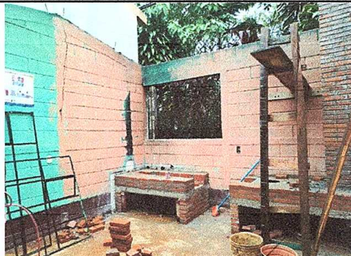
Foto 4: Reparación de cocina, sustitución de plancha y chimenea.
